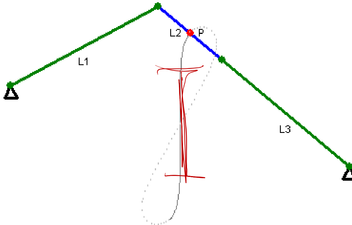
Mechanizm Watt'a
